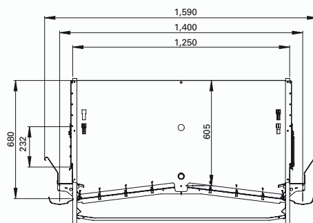
EV - P1250 鸡笼横截面 (不带风管)
