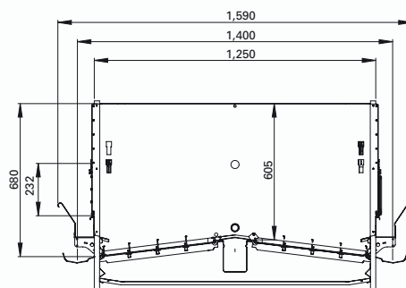
EV - P1250a 鸡笼横截面 (带风管)
